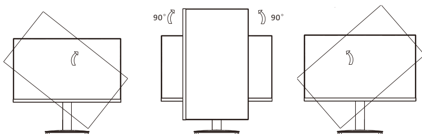
Angolo di rotazione della testa del monitor: -90^{\circ} \sim +90^{\circ}
