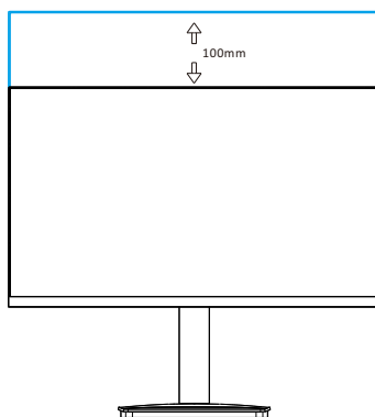
Regolazione dell'altezza della testa del monitor: 0 \sim 100\text{mm}
