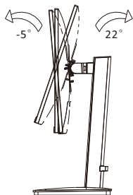
Angolo di inclinazione della testa del monitor: -5^{\circ} \sim 22^{\circ}
