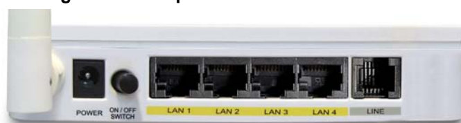
Figura 1. Vista posteriore del Router ADSL2+
